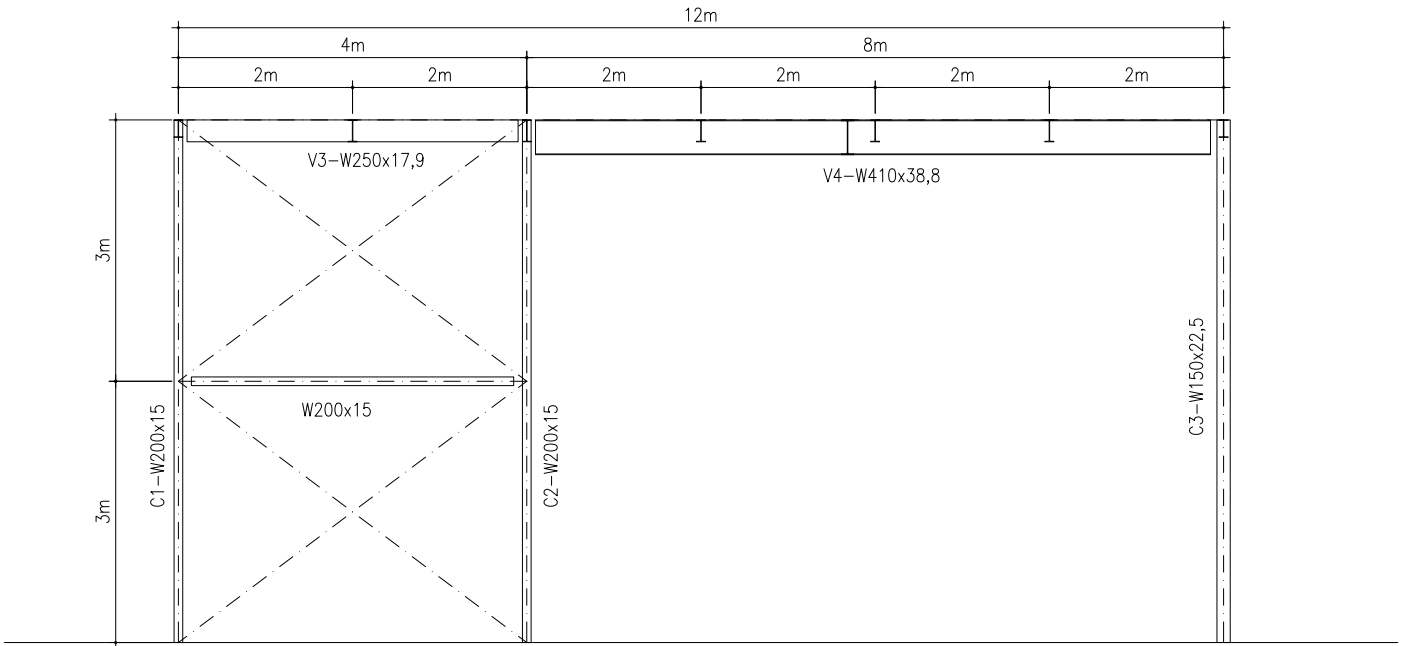
VISTA A-A
