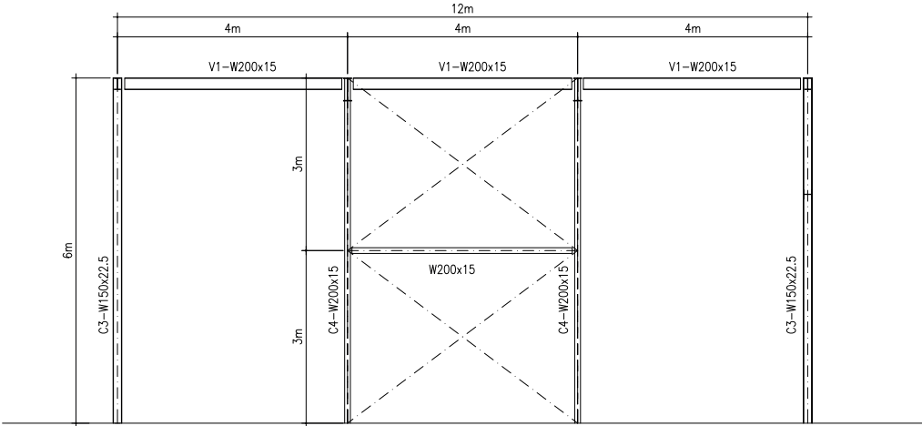
VISTA C-C
