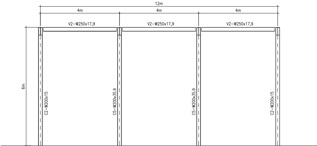
VISTA D-D
