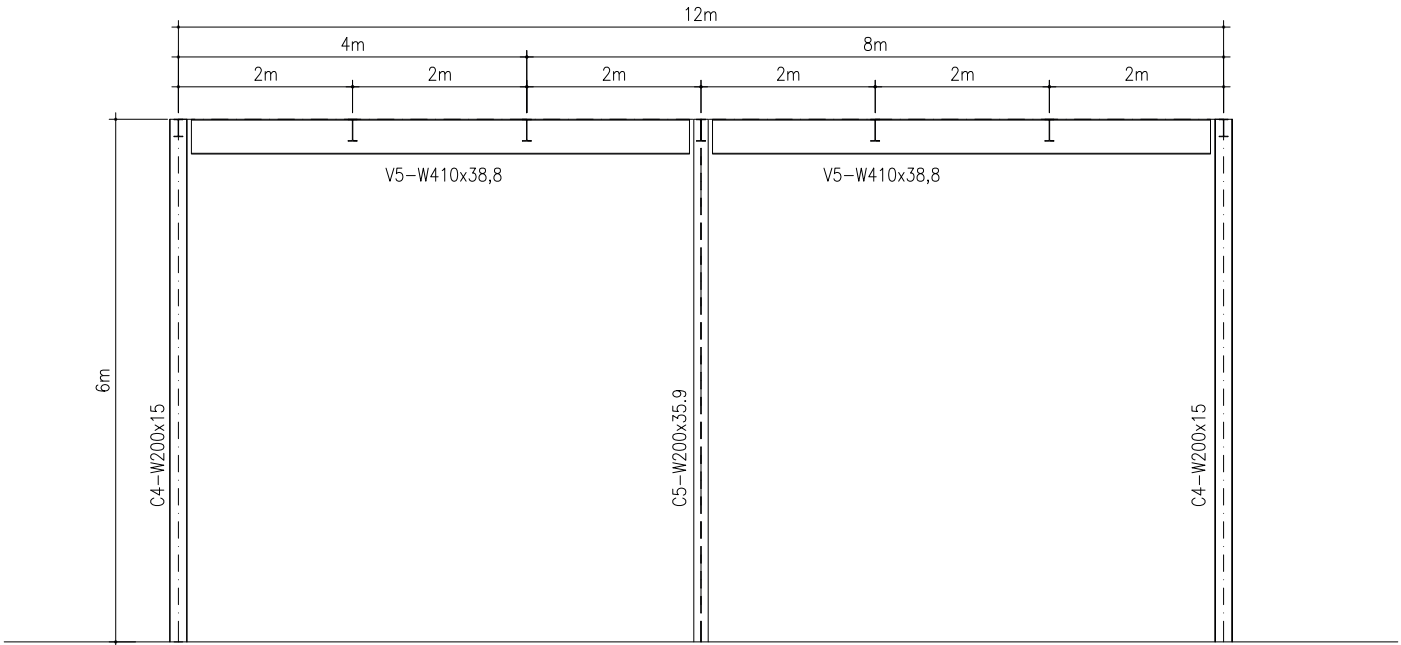
VISTA B-B
